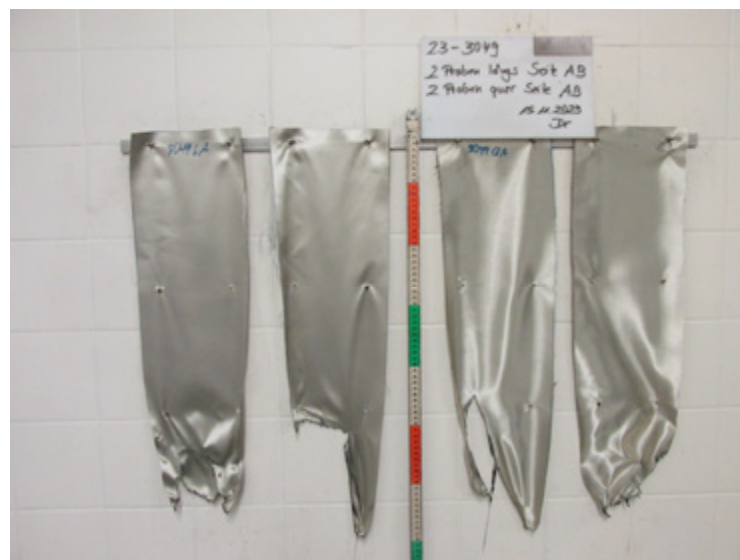
Bild 2: Aussehen der Proben nach dem Brandversuch
